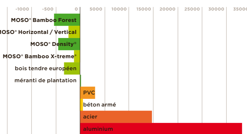
empreinte écologique sur l'ensemble du cycle de vie (kg CO2 eq/m³ matériaux)
